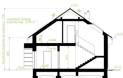
PRZEKRÓJ SKALA 1:100 PA - 10 0 0.5 1 1.5 2 2.5m
