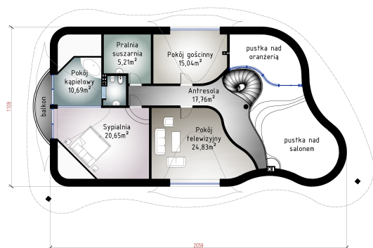
Rzut poddasza 94,18m 2
