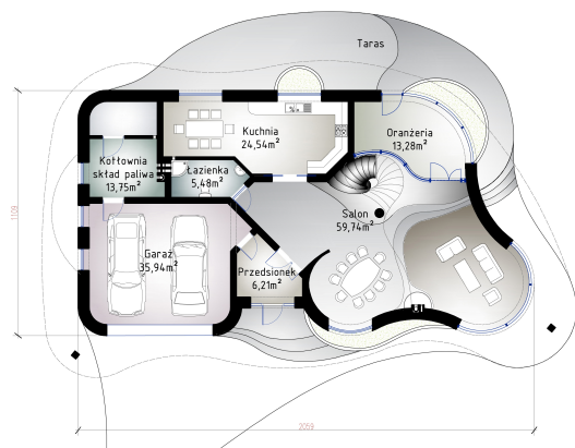
Rzut parteru 158,94 m 2
