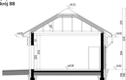
HomeKONCEPT-G 03 wersja podstawowa Przekrój BB
