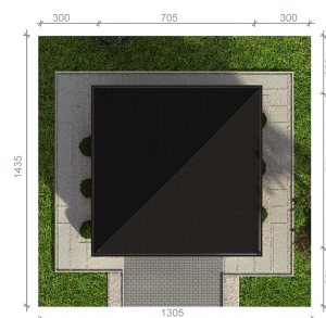
HomeKONCEPT-G 03 wersja podstawowa zagospodarowanie terenu
