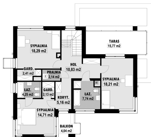
E-137 PIĘTRO
