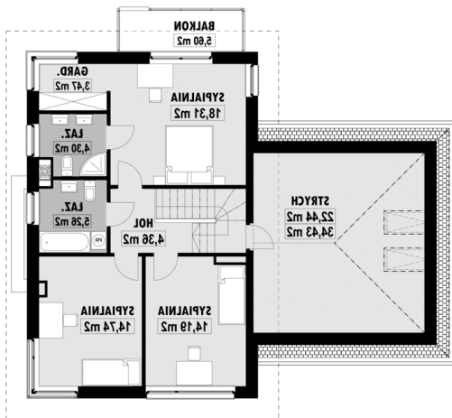
E-125 PIĘTRO
